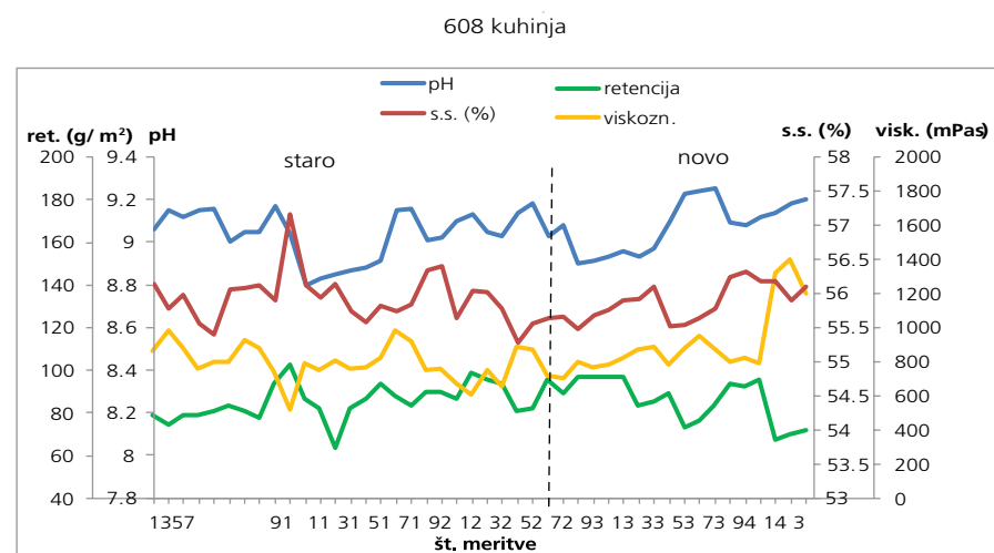
Figure 5: Prikaz vrednosti vodne retencije, pH, vsebnosti suhe snovi in viskoznosti za posamezne meritve. Otvzemno mesto: premazna kuhinja. Figure 5: Values for water retention, pH, dry content and viscosity for the individual measurements. Sampling spot: coating kitchen.
