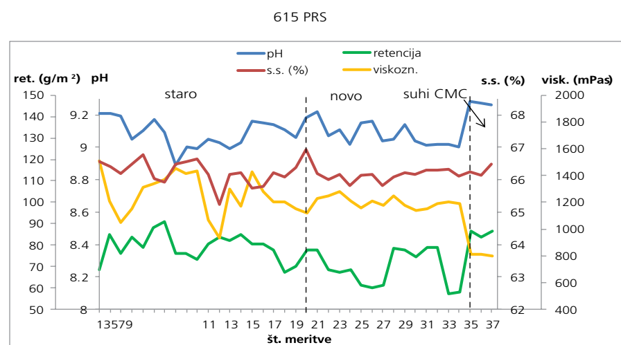
Slika 6: Prikaz vrednosti vodne retencije, pH, vsebnosti suhe snovi in viskoznosti za posamezne meritve. Otvzemno mesto: premazni stroj. Figure 6: Values for water retention, pH, dry content and viscosity for the individual measurements. Sampling spot: coating machine.
