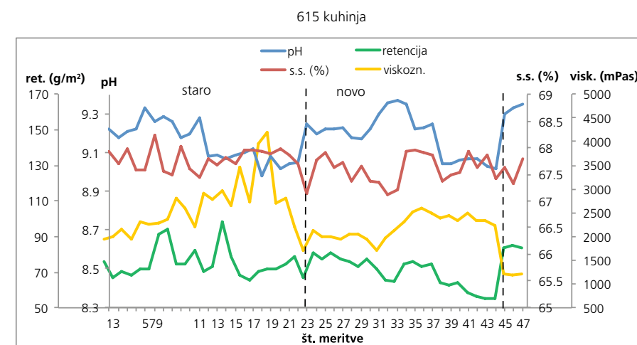
Slika 4: Prikaz vrednosti vodne retencije, pH, vsebnosti suhe snovi in viskoznosti za posamezne meritve. Odvzemno mesto: premazna kuhinja. Figure 4: Values for water retention, pH, dry content and viscosity for the individual measurements. Sampling spot: coating kitchen.
