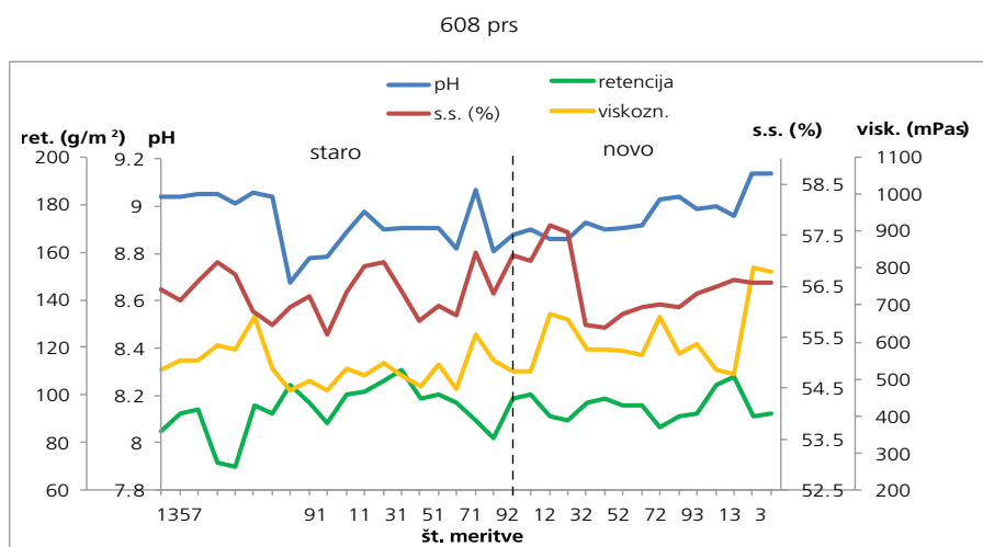
Slika 7: Prikaz vrednosti vodne retencije, pH, vsebnosti suhe snovi in viskoznosti za posamezne meritve. Otvzemno mesto: premazni stroj. Figure 7: Values for water retention, pH, dry content and viscosity for the individual measurements. Sampling spot: coating machine.
